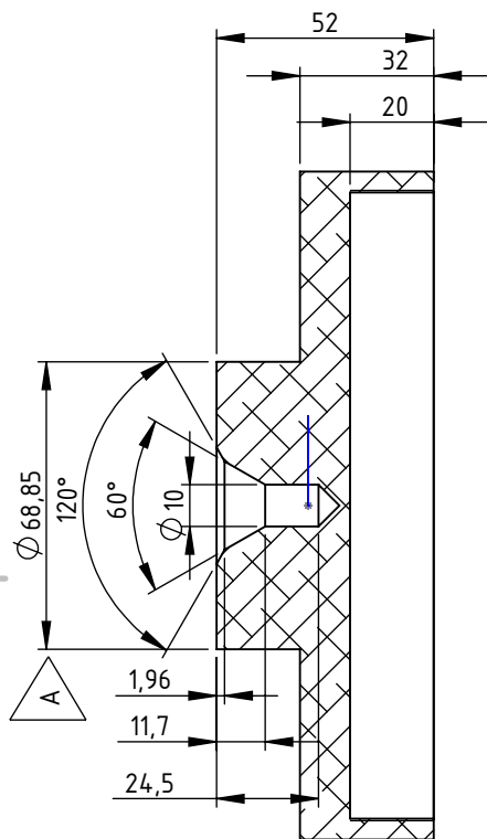
PRZEKRÓJ A-A
